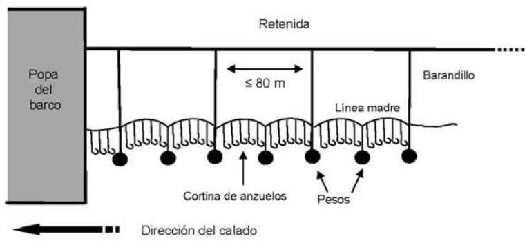
Configuración típica del sistema de palangre español
